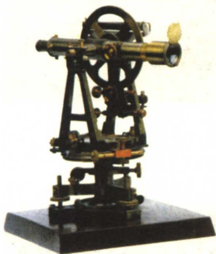
■ 铁路测量仪器
